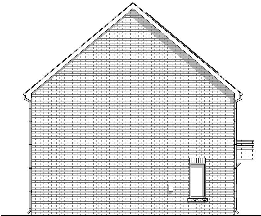
Left-Side Elevation
